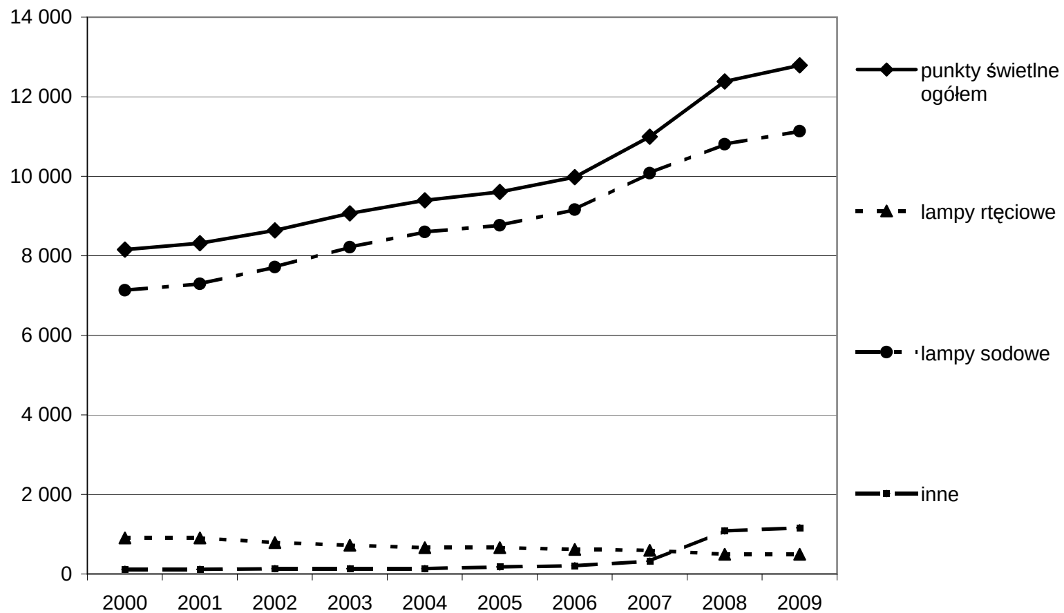
Wykres 7.1. Oświetlenie w Płocku w latach 2000 - 2009
